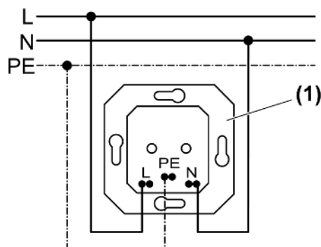
Bild 2: Anschlussplan Einzelsteckdose
