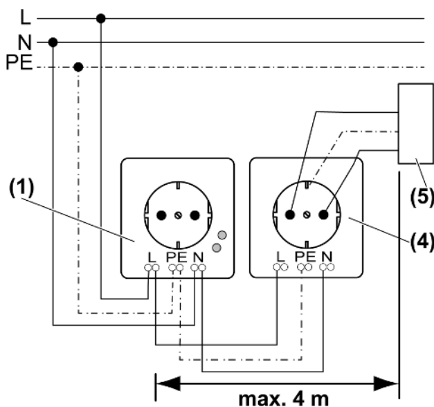
Bild 3: Anschlussplan Steckdosenkombination
