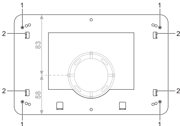
Abb. 2: Montage Adapter
