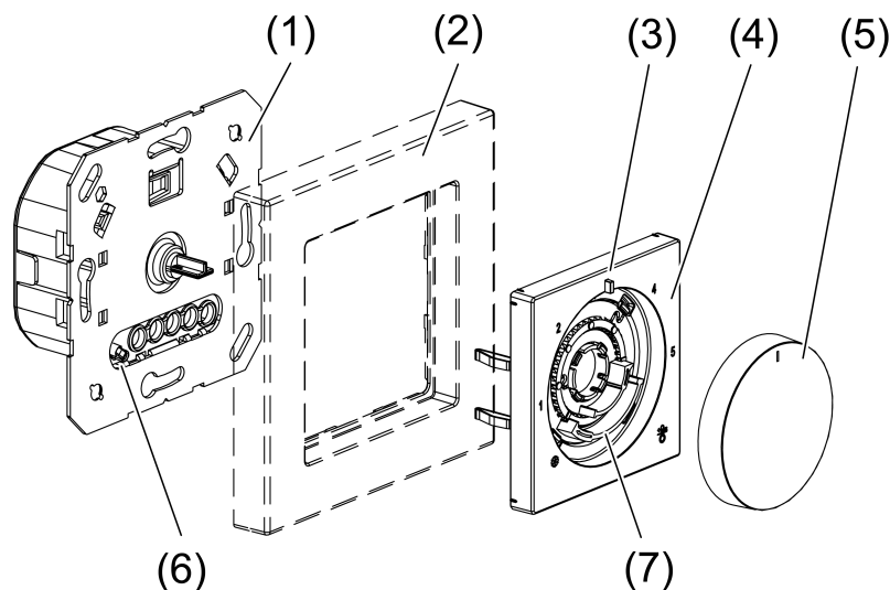
Bild 1: Geräteaufbau
