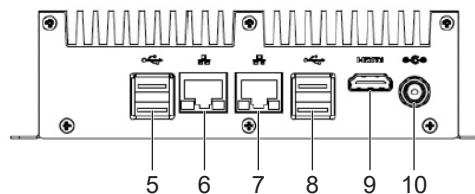
Abb. 2: Gerät Rückseite
