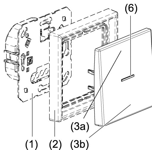
Bild 2: eNet Taster Standard
