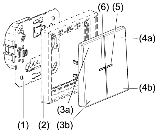
Bild 1: eNet Taster Universal
