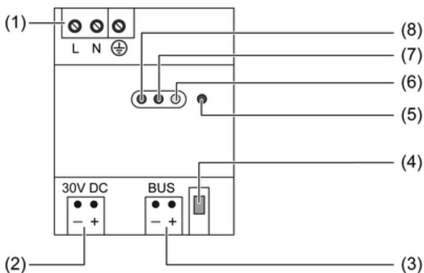
Bild 1: Spannungsversorgung 320 mA
