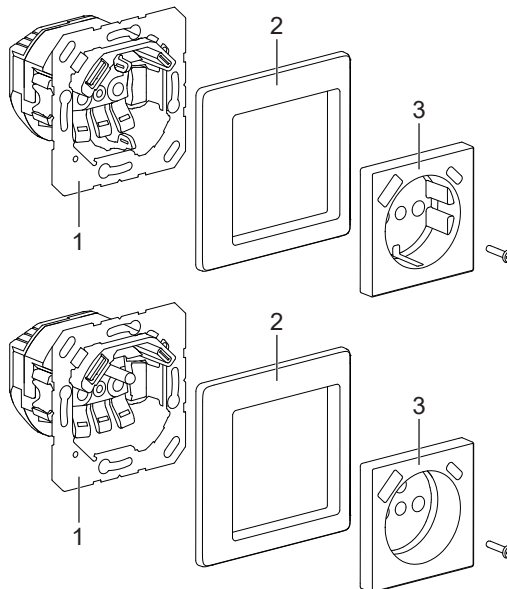
Abb. 1: Geräteaufbau
